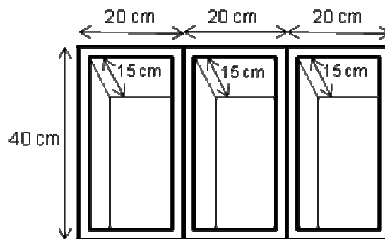
Figura 21 – Formas de madeira para a construção do tijolo de adobe
