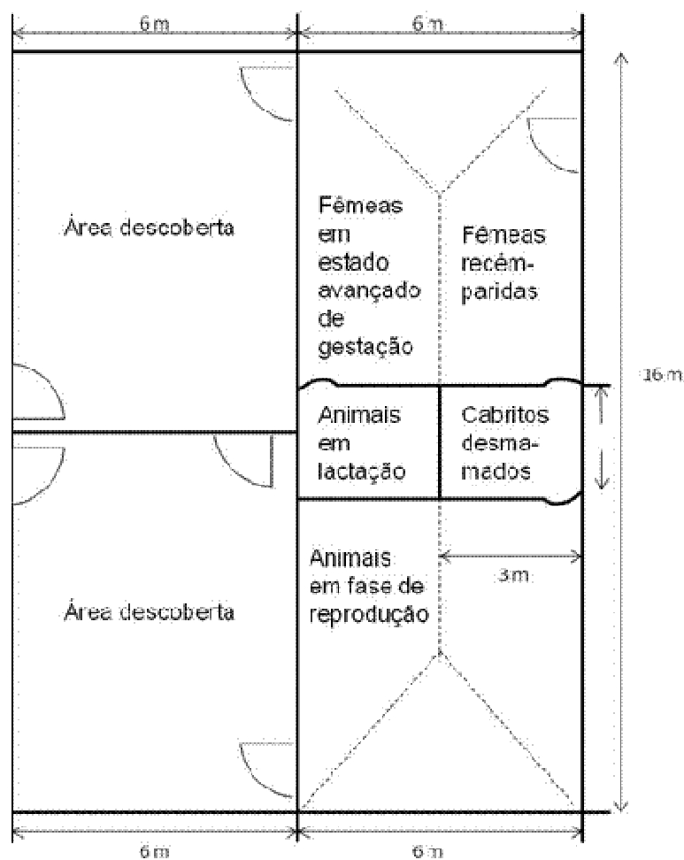
Figura 37 – Planta baixa do modelo de aprisco FONTE: Adaptado de SEBRAE/EMBRAPA (2003)
