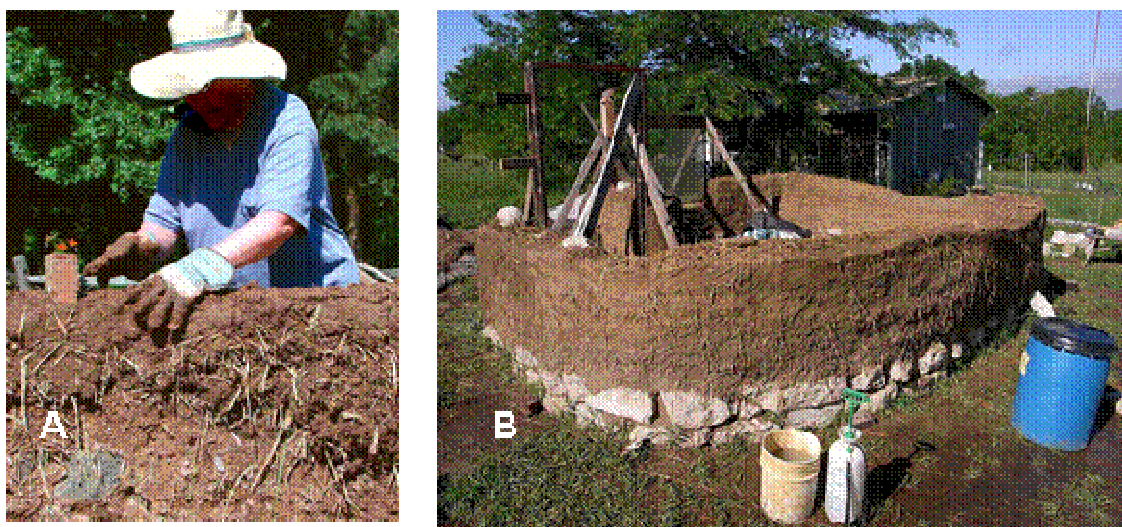
Figura 31 – Construção em COB. (a) Detalhe de parede sendo construída, (b) Observar a ausência de madeirame para a sustentação e as paredes curvas.
