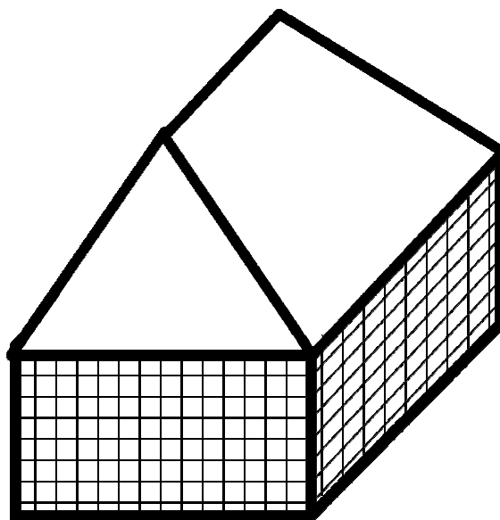
Figura 17 – Estrutura base da construção de uma casa de taipa de mão. FONTE: Adaptado de Brasil (2008)
