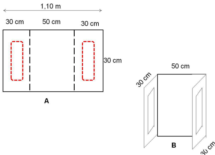
Figura 35 – Esquema de preparação da placa de sustentação da argamassa no revestimento interno da cisterna
