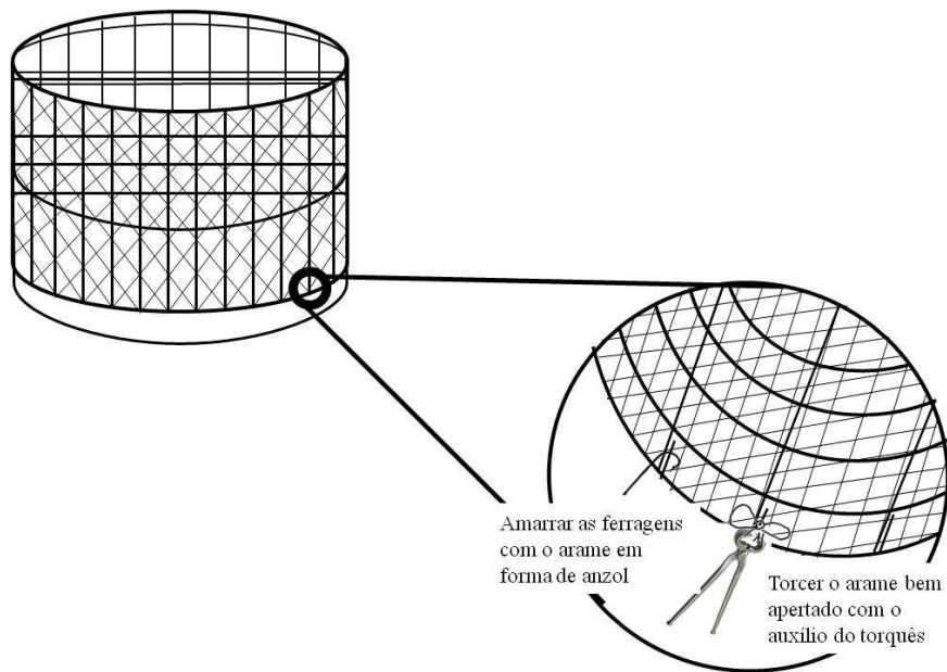
Figura 34 – Esquema de amarração da gaiola da cisterna na parte do piso que ficou dobrada para cima
