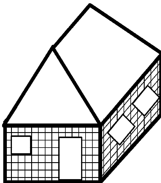
Figura 18 - Estrutura base da construção de uma casa de taipa de mão, com o lugar das portas e janelas. FONTE: Adaptado de Brasil (2008)
