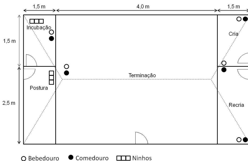
Figura 39 – Planta baixa do galpão do galinheiro com cinco divisões FONTE: Adaptado de EMBRAPA (2007)
