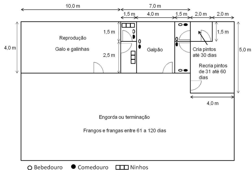
Figura 38 – Planta baixa dos piquetes do galinheiro FONTE: Adaptado de EMBRAPA (2007)
