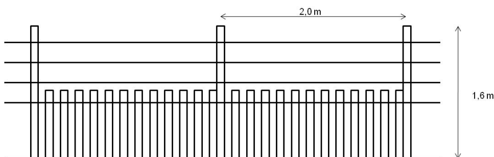
Figura 40 – Modelo de cerca com estacas, estacotes e arame para galinheiro FONTE: Adaptado de EMBRAPA (2007)
