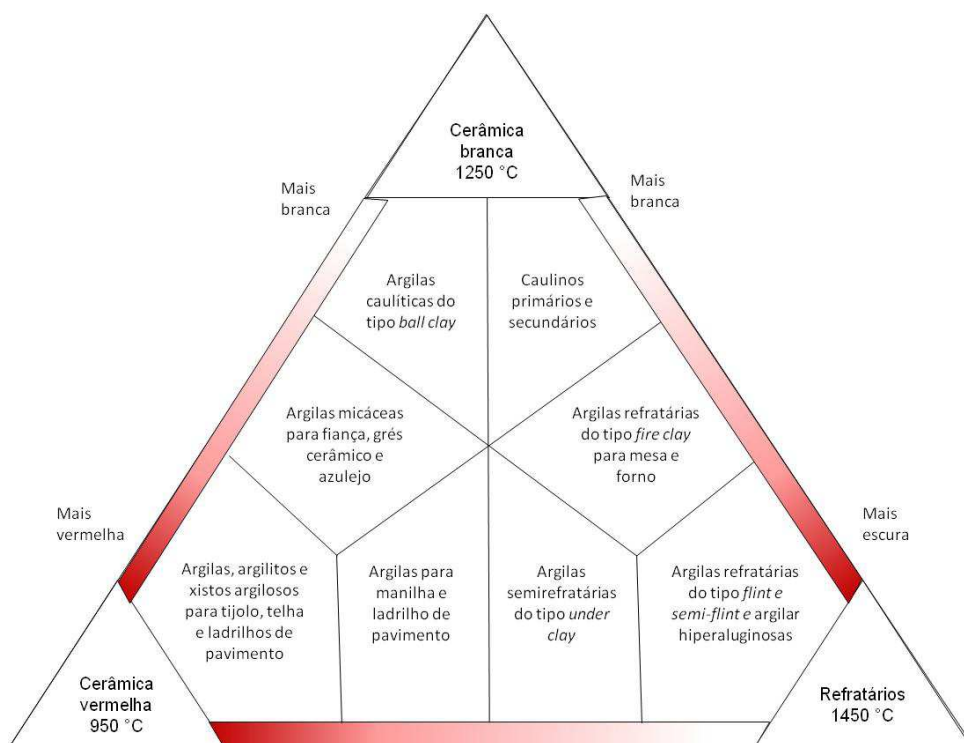
Figura 1 – Classificação das cerâmicas com base na cor após queima
