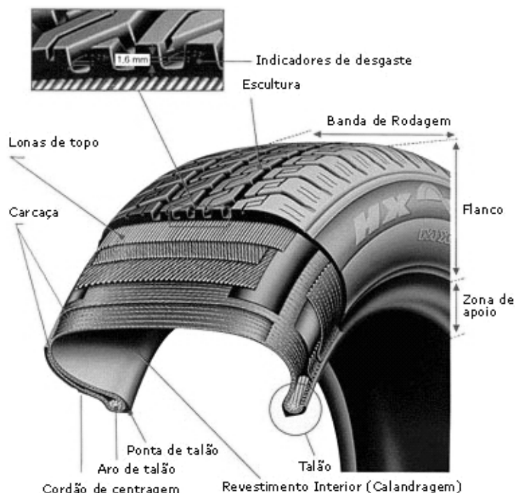
Figura 14 – Estrutura de um pneu radial (veículo de passeio)
