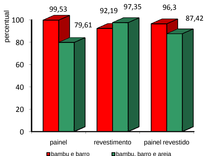
Gráfico 1 – Percentual de redução de custo na construção de painéis de barro comparada ao custo de alvenaria, chapisco e massa única 7 FONTE: Adaptado de Carvalho e Silva (2007)
