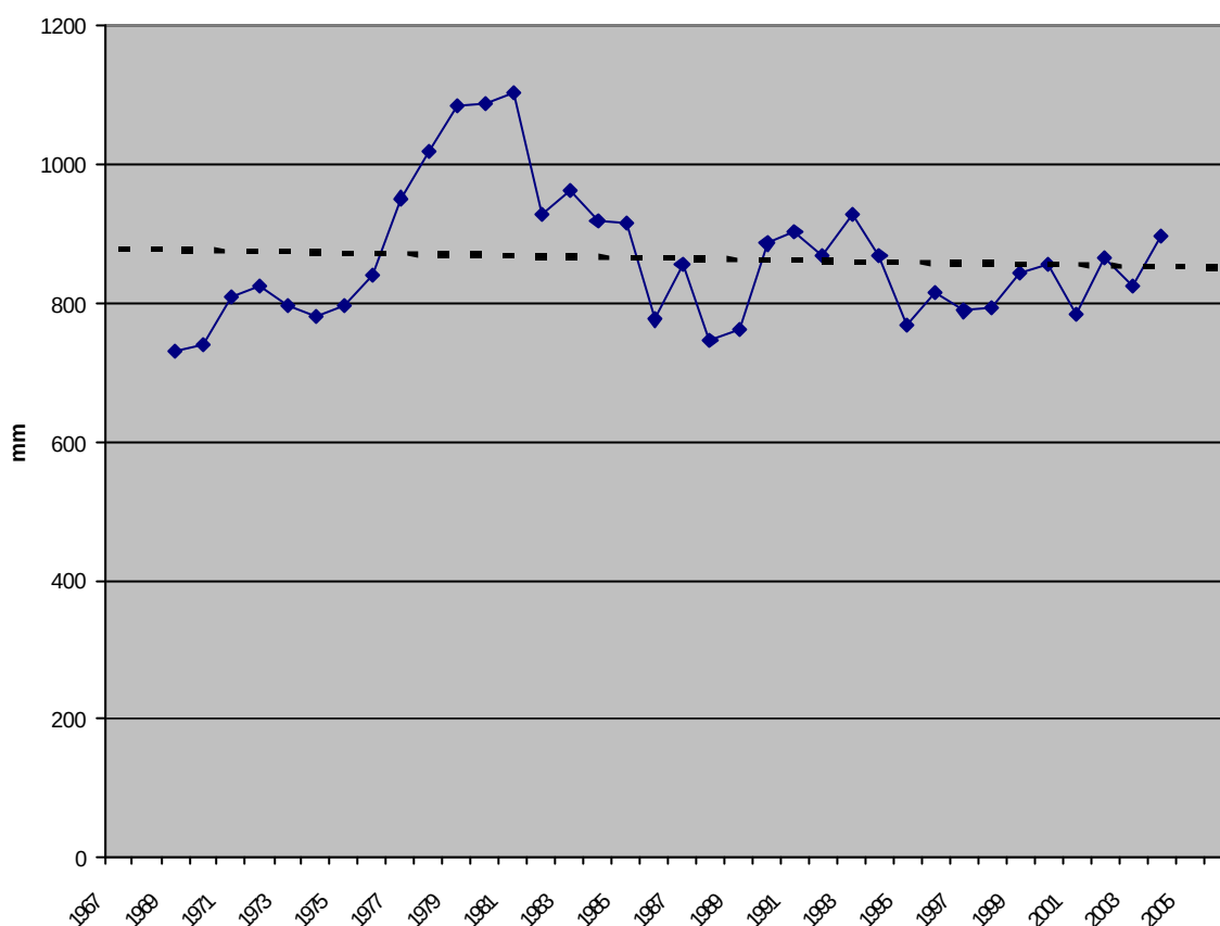
Gráfico 8 – Média móvel da precipitação pluviométrica anual na cidade de Salinas-MG, no período de 1967 a 2006.
