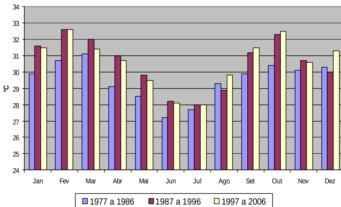
Gráfico 4 - Temperatura média das máximas na cidade de Salinas-MG, em cada década do período de 1977 a 2006.
