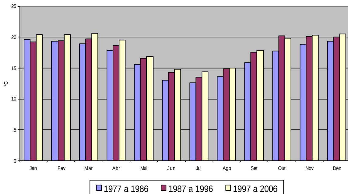
Gráfico 5 - Temperatura média das mínimas na cidade de Salinas-MG, em cada década do período de 1977 a 2006.
