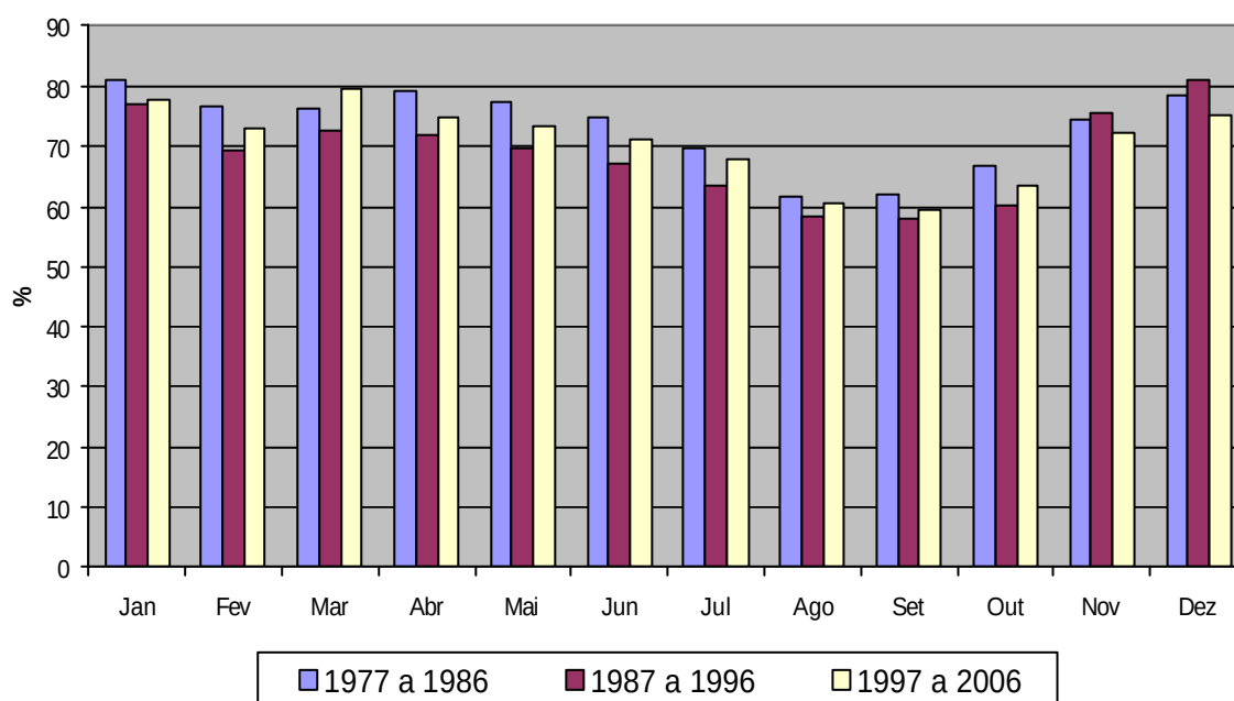
Gráfico 6 – Média diária da umidade relativa do ar, na cidade de Salinas-MG, em cada década do período de 1977 a 2006.
