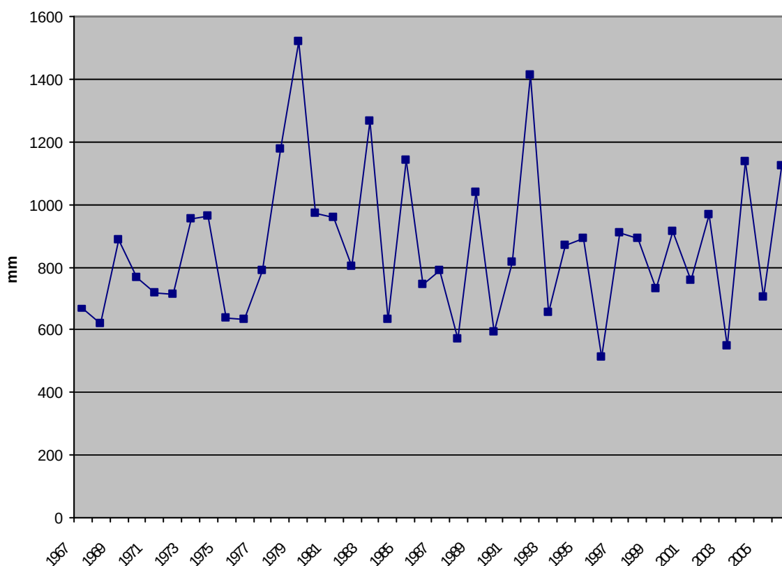
Gráfico 7 – Precipitação pluviométrica anual na cidade de Salinas-MG, no período de 1967 a 2006.
