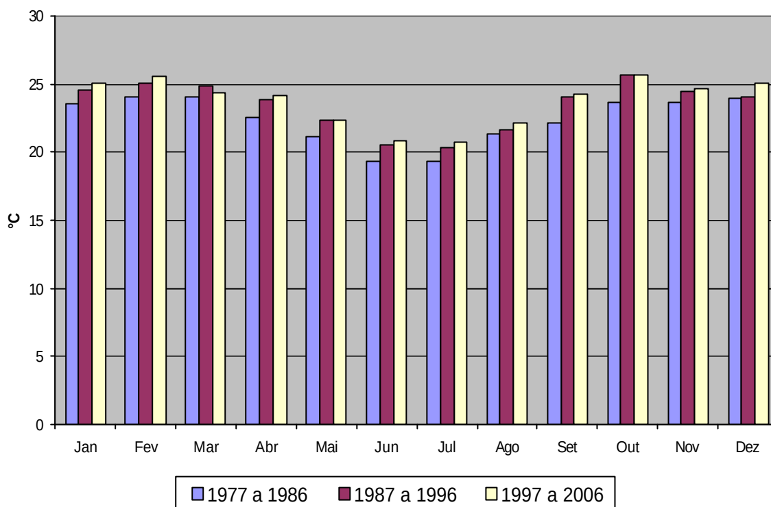
Gráfico 3 – Temperatura média compensada na cidade de Salinas-MG, em cada década do período de 1977 a 2006.
