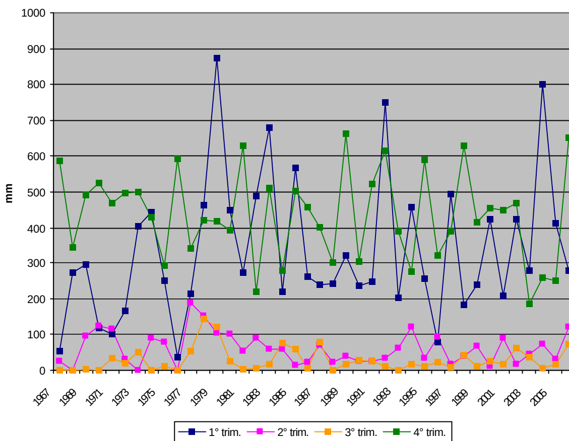
Gráfico 10 – Precipitação pluviométrica trimestral na cidade de Salinas, no período de 1967 a 2006.
