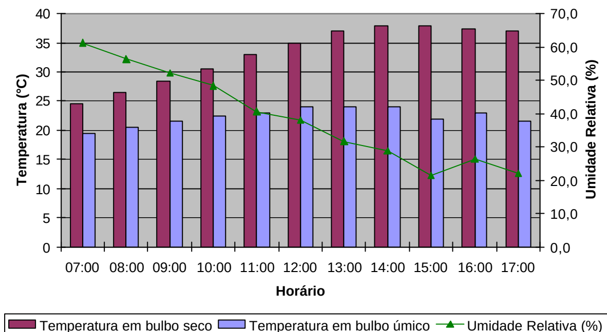
Gráfico 1 – Temperatura e umidade relativa do ar em Salinas-MG, no dia 31 de outubro de 2008, de acordo com dados coletados em psirômetro.
