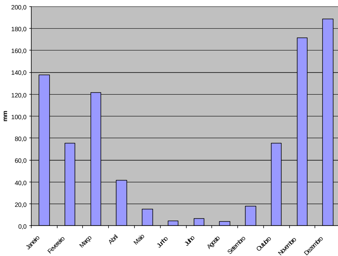
Gráfico 9 – Média da precipitação pluviométrica mensal na cidade de Salinas-MG, no período de 1967 a 2006.
