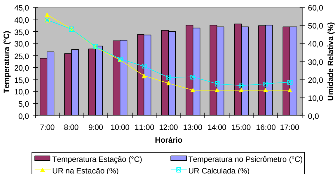
Gráfico 2 – Comparação entre os valores de temperatura e umidade relativa do ar obtidas por Estação Automatizada e por psicrômetro sem ventilação forçada.
