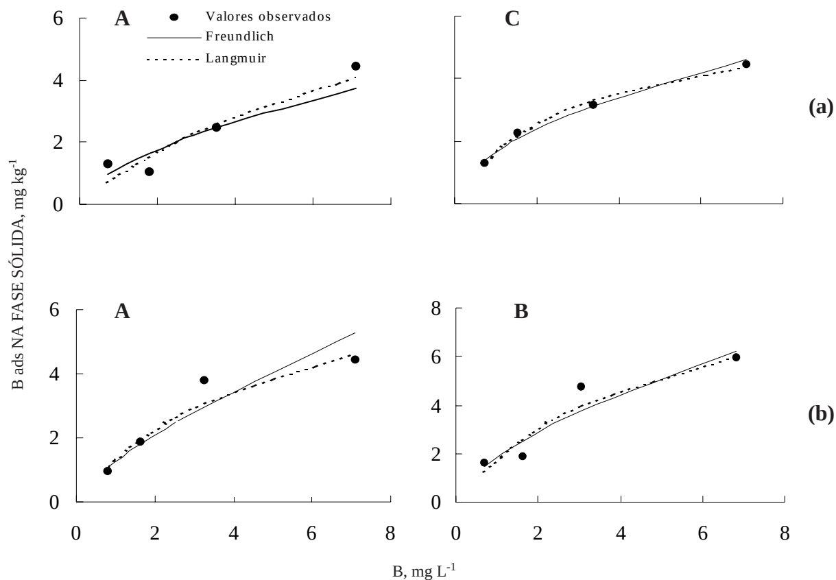
Figura 1. Isotermas de adsorção calculadas pelos modelos de Freundlich e de Langmuir e seus dados obtidos experimentalmente, para as amostras de superfície e subsuperfície de um Glei Pouco Húmico A e C (a) e de um Cambissolo distrófico A e B (b).
