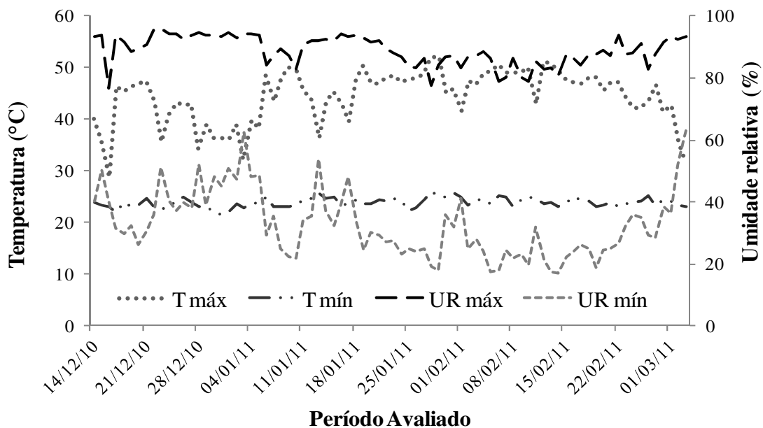
Figura 10. Variações de umidade relativa do ar e oscilações de temperatura registradas pelo termohigrógrafo no interior da casa de vegetação.
